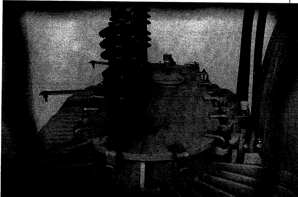
Figura 1 – Marcas de vazamento de óleo na base do isolador.
