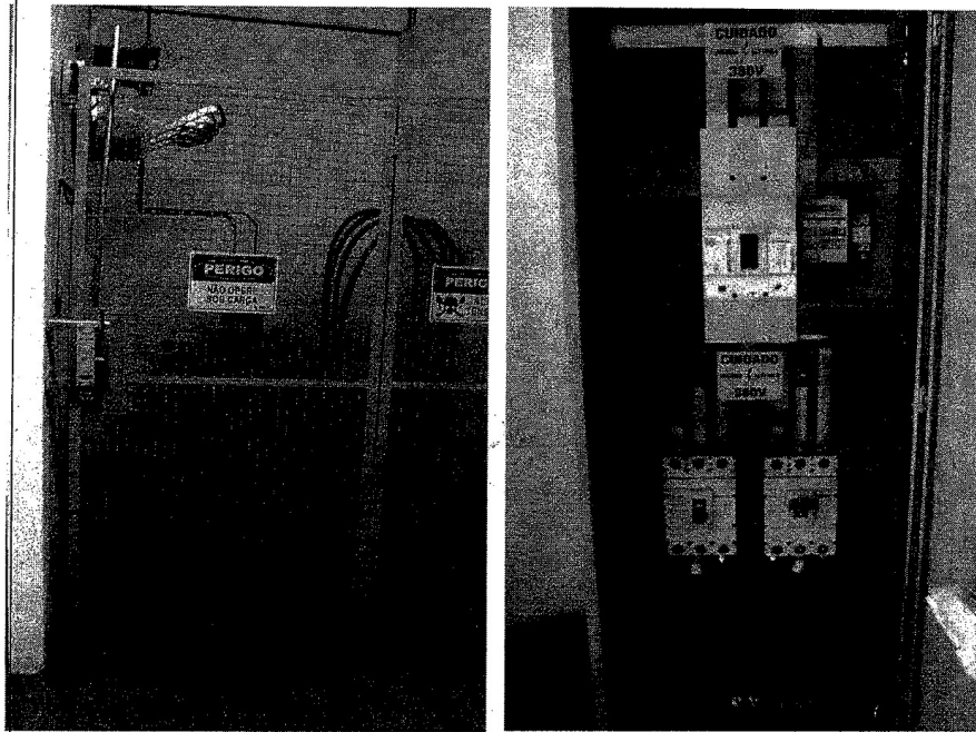
Figura 2 – a) Marcas de vazamento de óleo no cubículo do transformador. b) Disjuntores Gerais do QGBT, disjuntor do transformador avariado está desligado.
